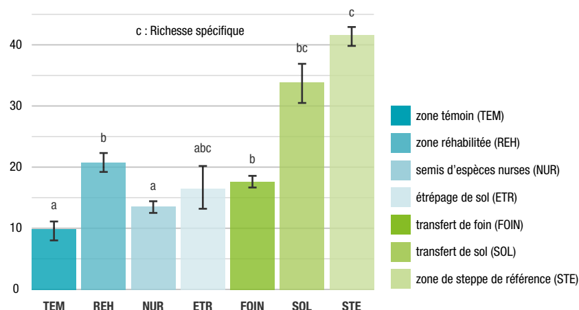
Figure 2 : Richesse spécifique en fonction des traitements de restauration : Au sein de chaque graphique, deux bars surmontées par une lettre identique ne présentent pas de différences significatives.
